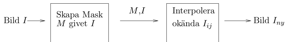
Figur 1: Bildbehandlingsproblem löses genom att man först skapar en mask M som talar om vilka platser i I matrisen som skall betraktas som okända. I interpolationssteget beräknas lämpliga värden på de okända pixlarna I_{ij} .
